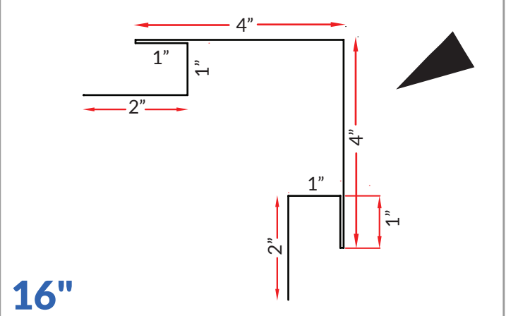
7/8 OSC 4 x 4
