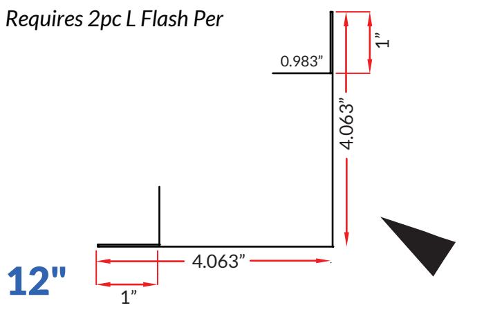
7/8 3PC OSC CAP 4 x 4
